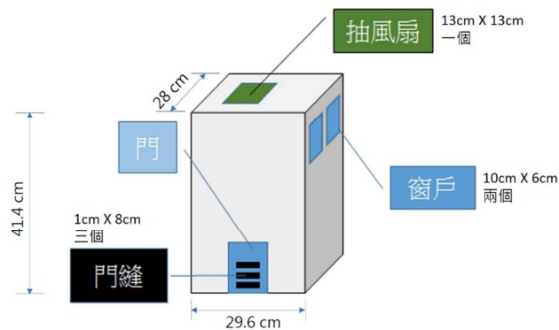
圖三：浴室模擬箱
