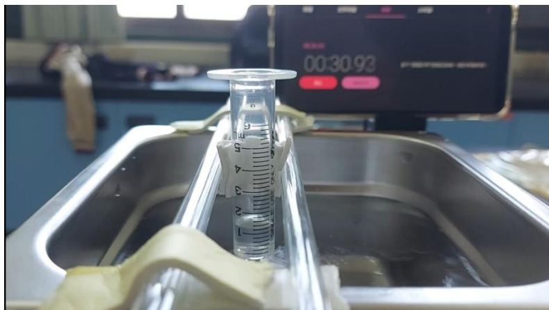
圖 4、實驗照片
